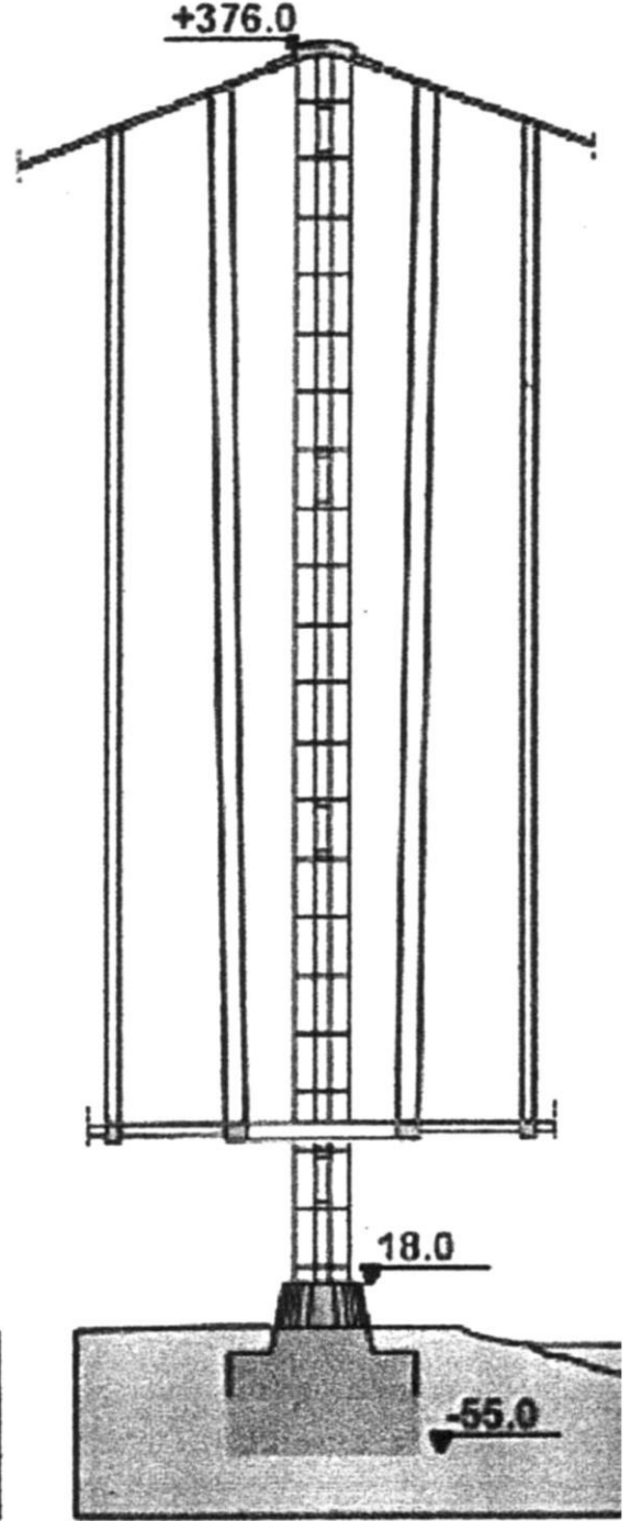
VISTA LONGITUDINALE
