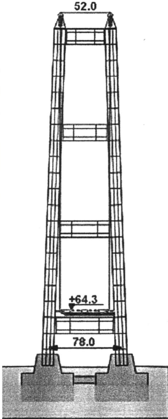
VISTA TRASVERSALE
